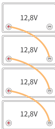
Reihenschaltung 48V(51,2V) 45Ah
